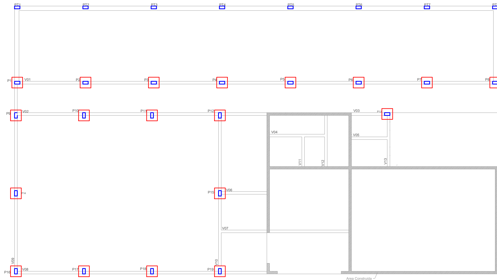
PLANTA ESTRUTURAL ESC: 1/75
