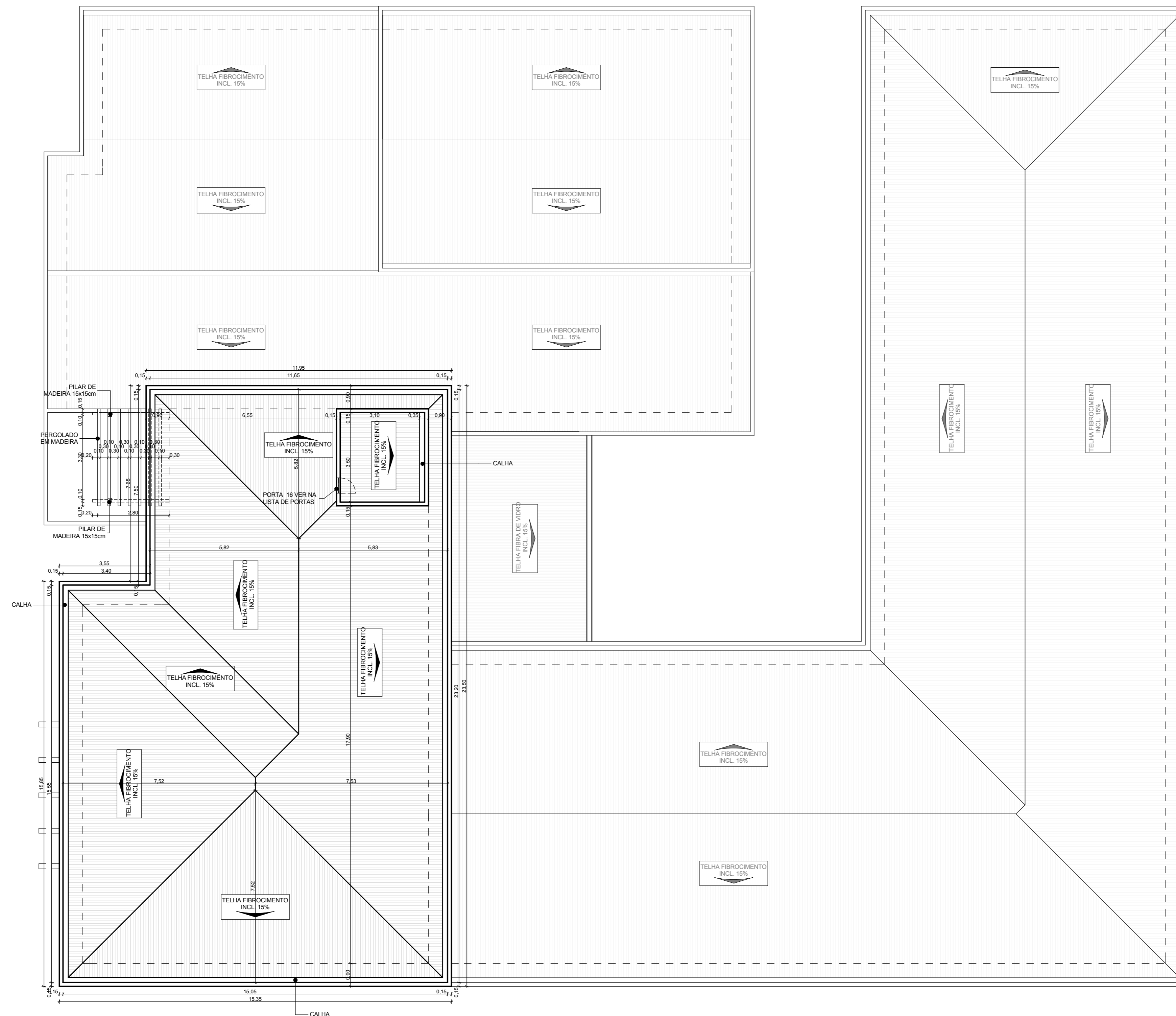
COBERTURA ESCALA.: 1/100
