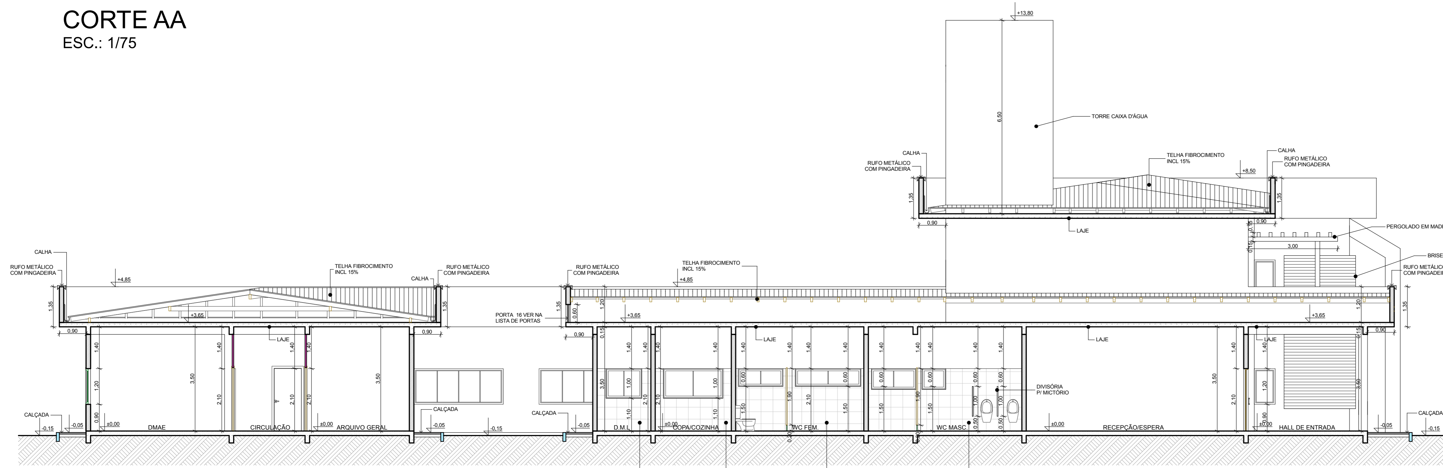
CORTE BB ESC.: 1/75
