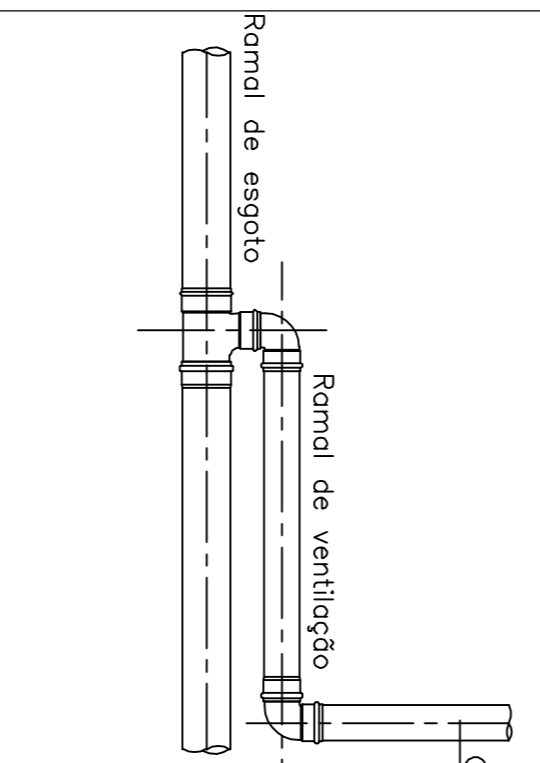
DETALHE ESCOVA DE LIGAÇÃO DO RANHAL E COLUMNA DE VENTILAÇÃO
