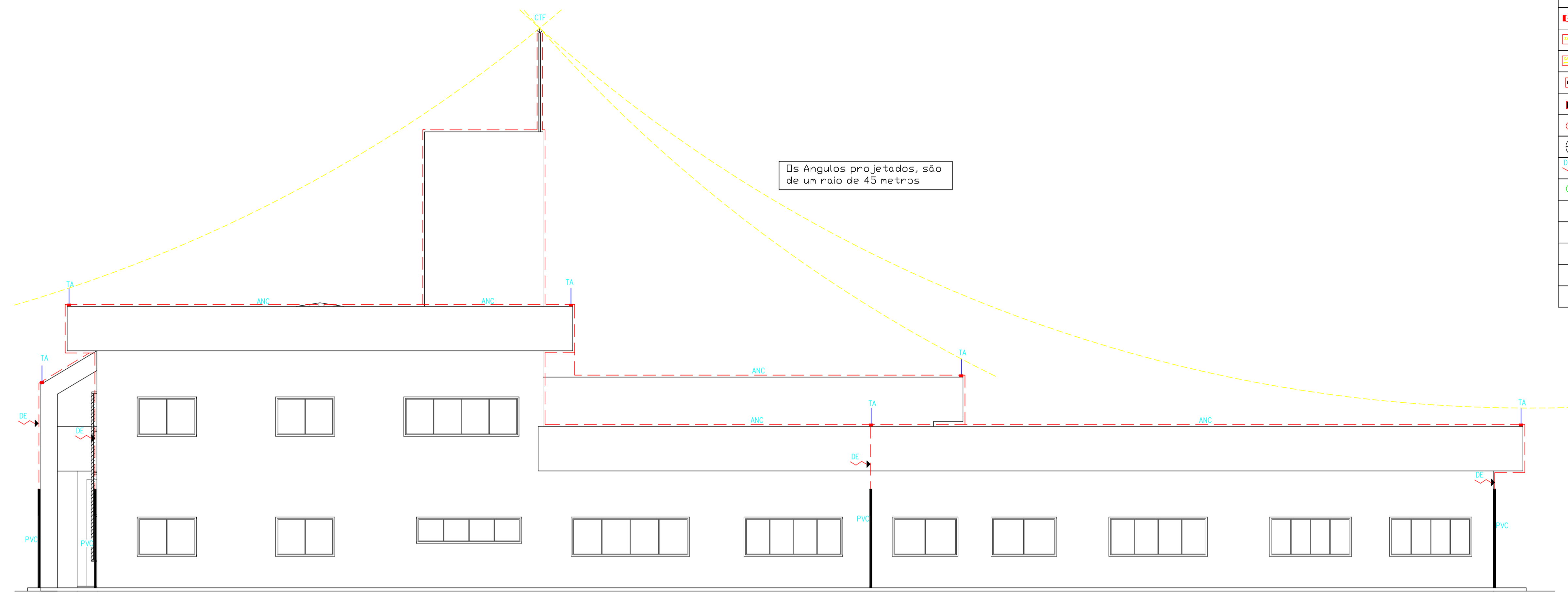
VISTA 04 ESC.: 1/75
