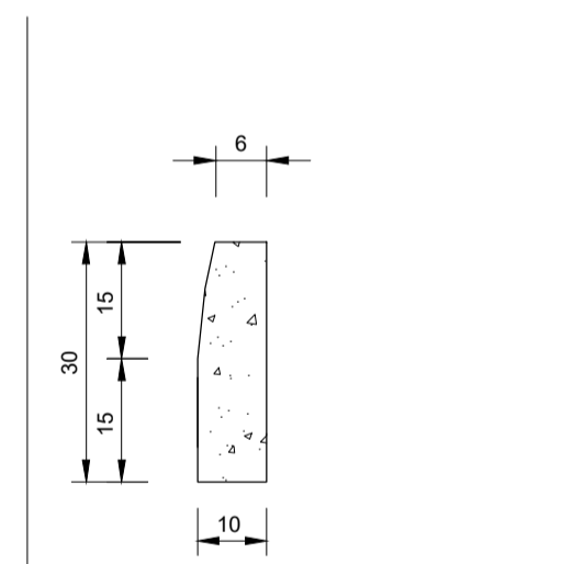
03 Detalhe Meio Fio Tipo 01 Esc.: 1/10 Meio fio
