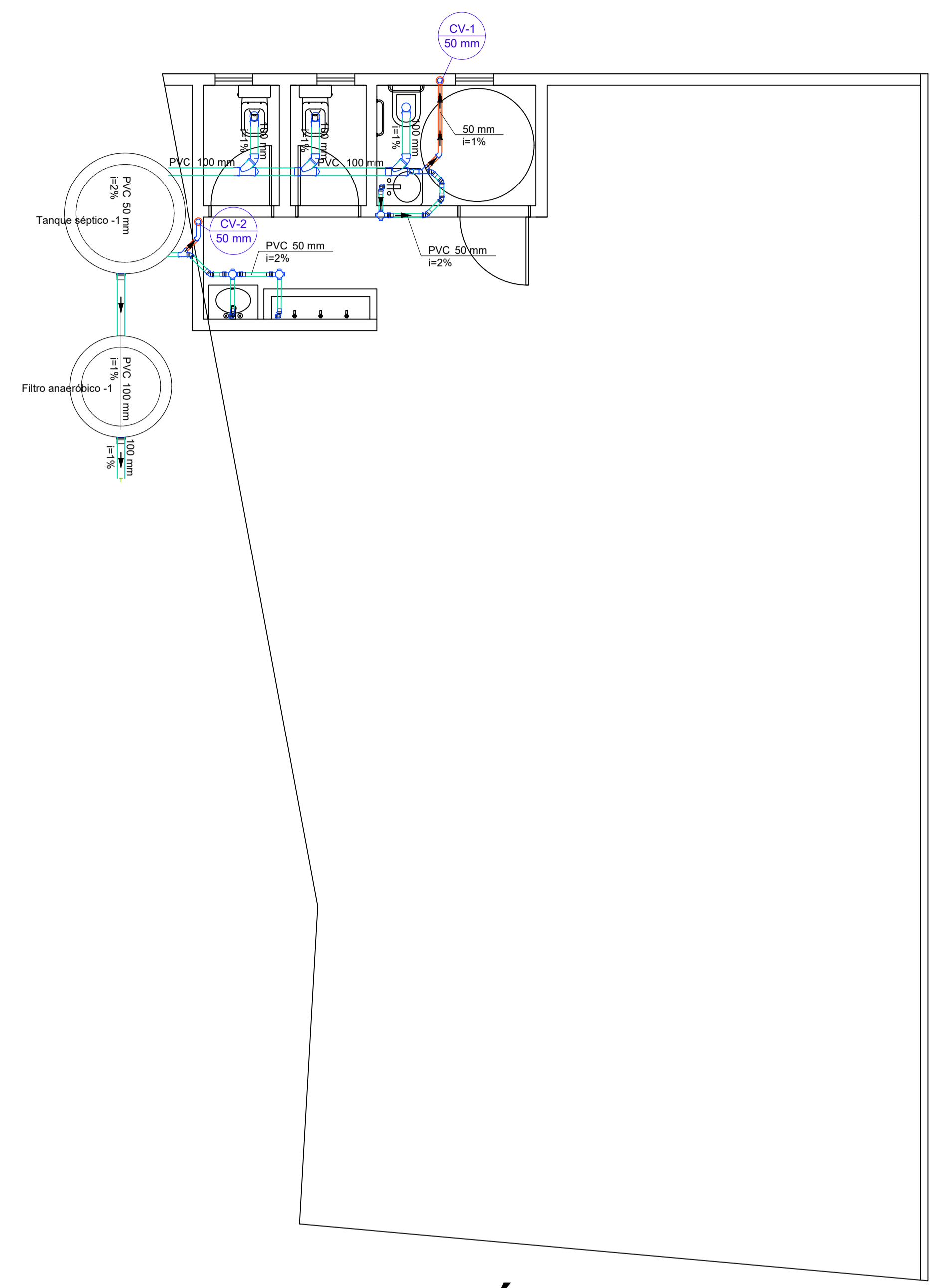
SANITÁRIO esc 1:50
