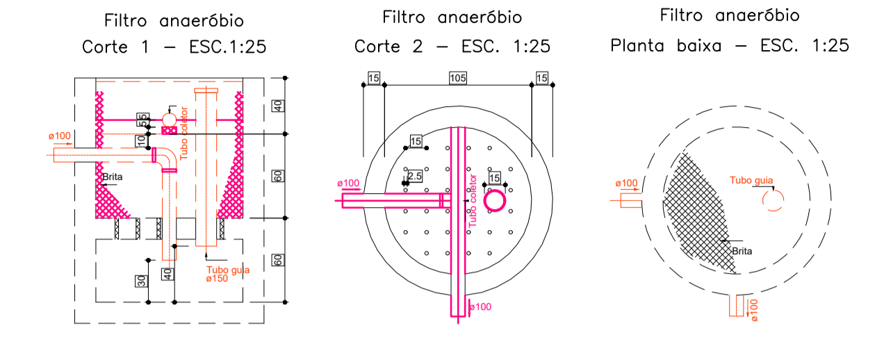
DETALHE FILTRO ANEARÓBIO esc 1:50
