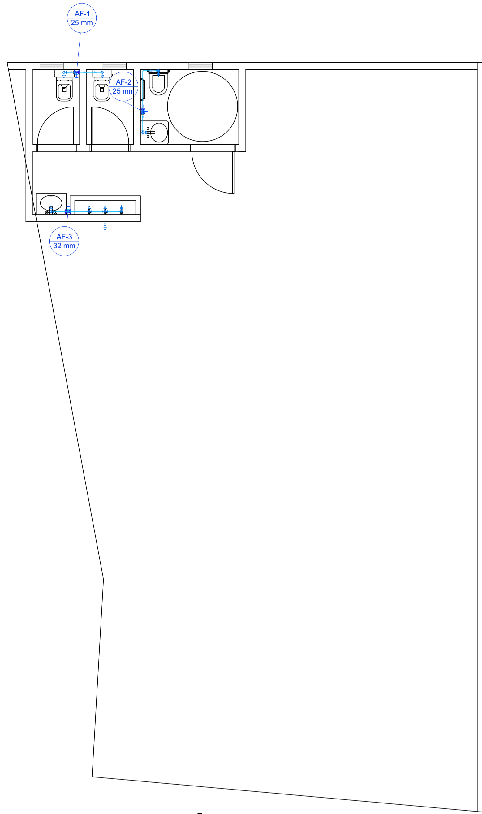
HIDRÁULICO esc 1:50
