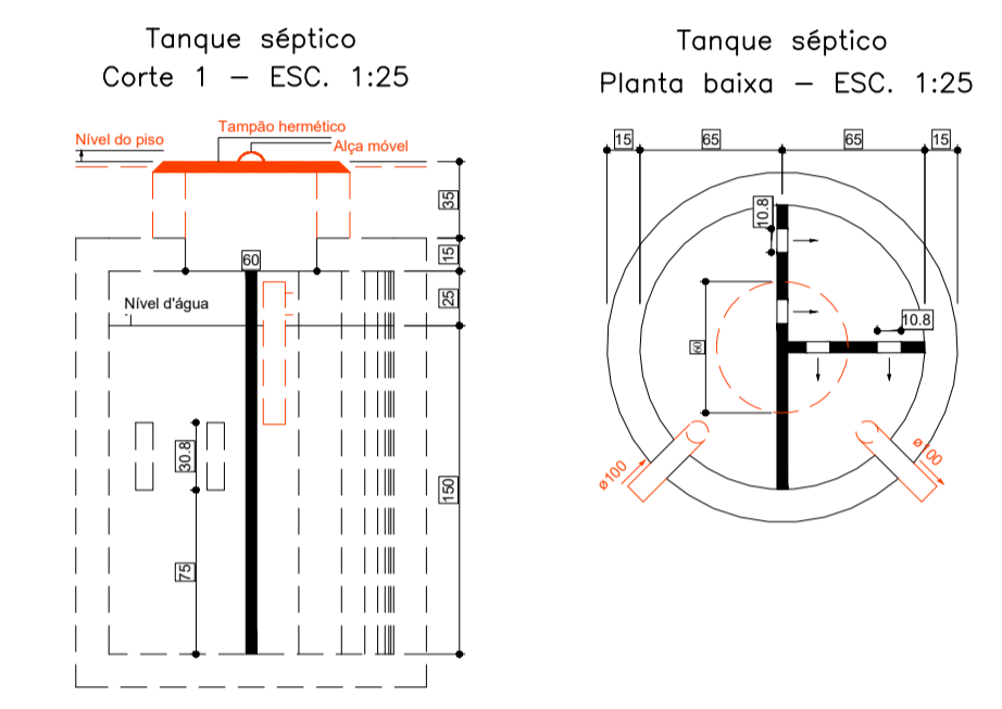
DETALHE TANQUE SÉPTICO esc 1:50
