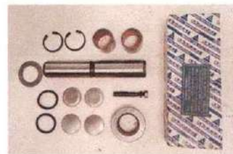
Embuchamento 1/2 Jogo C/ Rolamento Sm-35,40 Fp-1380r Fabraço
