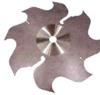
Serra 400mm x 8 Dentes + 2 Raspadores, Corte 5,5mm
