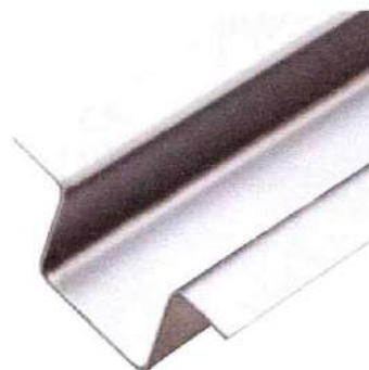
Perfil Cartola Aço SAE 30x27x15mm x 1,20mm x 3000mm
