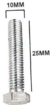
Parafuso sextavado 10 x 25mm ma zb aço 8.8
