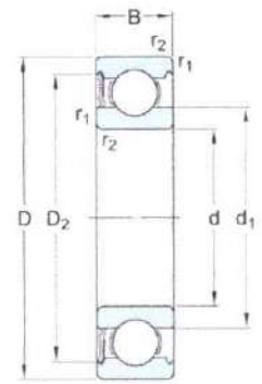
Rolamento Rigido De Esferas SKF 6204-Z/C3
