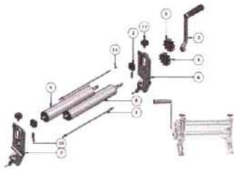
Engrenagem do Cilindro Manual Botini Direita e Esquerda Ferro
