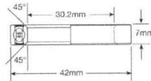
Rolamento Caixa De Direção Enduro 6806 Llb Osid (30.2x42x7: 45x1°) - Pinarello
