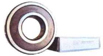
Rolamento 6307 Nsk Ddu 2rs C3 - 35x80x21mm - P/ Alta Rotação
