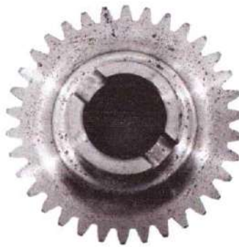
Engrenagem Do Cilindro Movel 34 Dentes Nogueira E Jf Cód 03.049265
