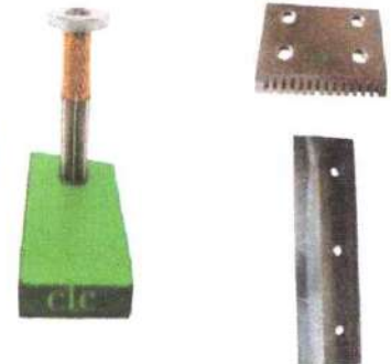
Rebolo Afiador P/ensiladeira Jf 92/z10 C120 (02.48715)
