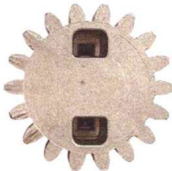
Engrenagem Externa Z18 P/ Motor Ppa Dz Predial Eixo 25mm
