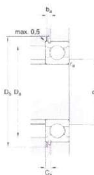
Rolamento Rígido De Esferas SKF 6307 NR/C3
